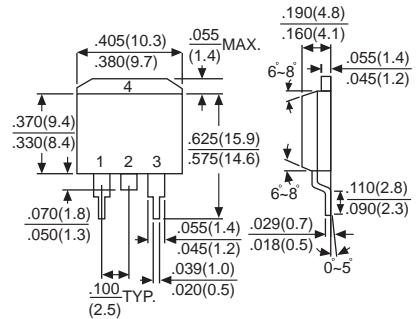
TO-263(D 2 PAK)
